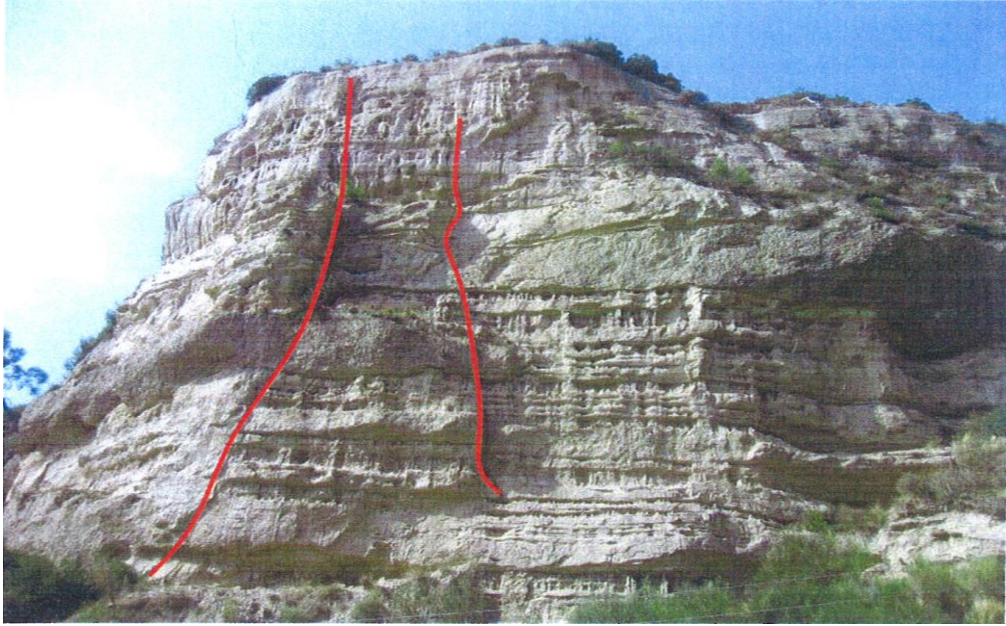
Φωτ. 17: Άποψη του απότομου πρανούς που δομείται από εναλλαγές ψηφιδωπαγών, φαμμιτών και ιλυολίθων. Παρατηρούνται οι εγκάρσιες ασυνέχειες και οι ρωγμές αποτόνωσης που δημιουργούν τα προβλήματα καταπτώσεων.[13]
