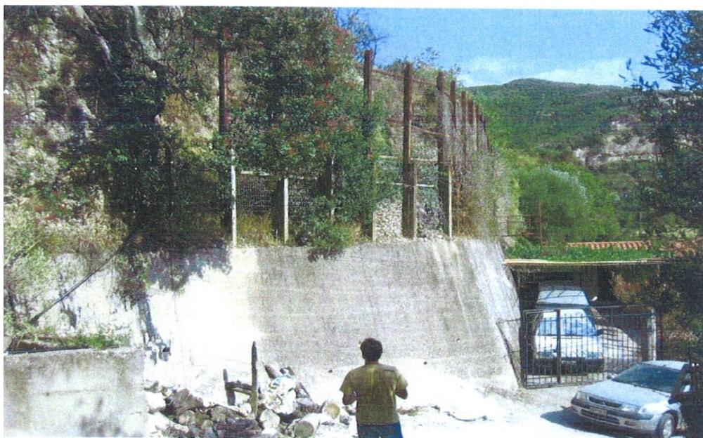
Φωτ. 19: Αποψη του μεταλλικού φράκτη που είχε κατασκευαστεί στο παρελθόν για την προστασία της οικίας από καταπτώσεις βράχων (θέση Α).[13]
