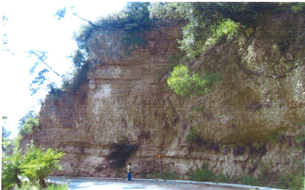
Φωτ. 14: Υψηλό και απότομο πρανές από κροκαλοπαγή. Είναι εμφανή τα προβλήματα πτώσεων τεμαχών και αποσαθρωμάτων στο οδόστρωμα, καθώς και η επικινδυνότητα πτώσης τεμαχών και στοιχείων της βλάστησης από υψηλότερες θέσεις.[13]
