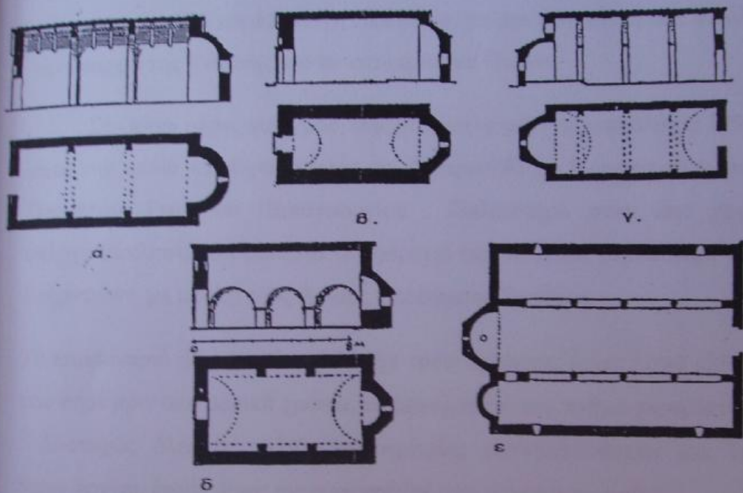
Κατώψεις και τομές βασιλικῶν τῆς Τουρκοκρατίας: α) ξυλοστεῖγου με ἐγκάρσια τόξα, β) ἀπλῆς καμαροσκεποῦς, γ) καμαροσκεποῦς με σφειδόνια, δ) καμαροσκεποῦς με πλευρικά τυφλά ἀψιδάματα, ε) τρικλίτου ξυλοστεῖγου (Α. Ὁρλάνδος).
