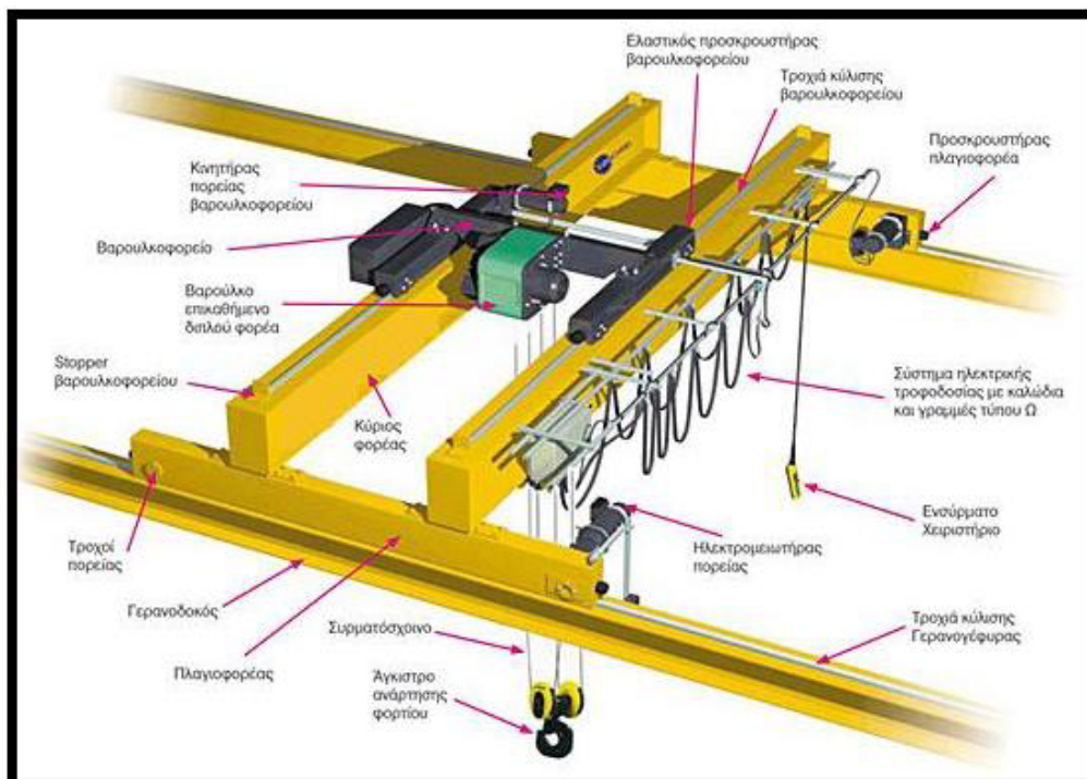
Σχήμα 5.1 Τυπική διάταξη γερανογέφυρας [4].
