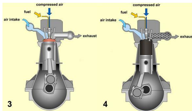
Σχήμα 6.2. Φάσεις ανάφλεξης- εκτόνωσης και εξαγωγής. [29]
