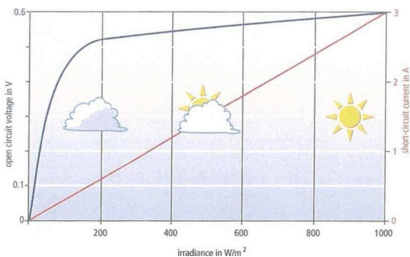
Σχήμα 3.10. Η μεταβολή της ανοιχτοκυκλωμένης τάσης V_{oc} (μπλε καμπύλη) και της βραχυκυκλωμένης έντασης I_{sc} του ρεύματος (κόκκινη καμπύλη) ενός \Phi/B στοιχείου πυριτίου σε συνάρτηση με την ισχύ της ακτινοβολίας H , που δέχεται ανά μονάδα επιφάνειάς του.
