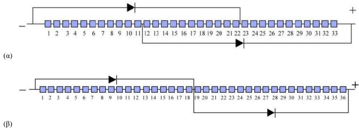
Σχήμα 3.19. (α) στοιχεία που επικαλύπτονται και (β) στοιχεία που δεν επικαλύπτονται.
