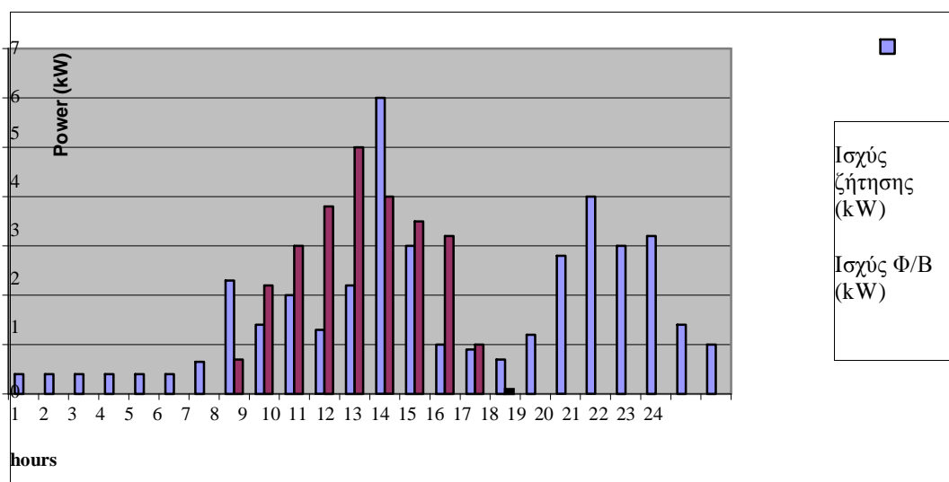
Σχήμα 7.8. Συγκριτικό ιστόγραμμα παραγόμενης ισχύος πλαισίων και καταναλισκομένης ισχύος από οικιακές συσκευές για κάθε ώρα ημέρας Δεκεμβρίου.
