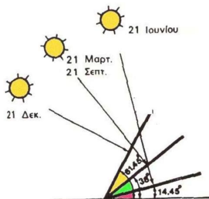
Σχήμα 2.16. Η βέλτιστη κλίση ενός ηλιακού συλλέκτη στο θερινό (21 Ιουνίου) και το χειμερινό (21 Δεκεμβρίου) ηλιοστάσιο και στην εαρινή (21 Μαρτίου) και τη φθινοπωρινή (21 Σεπτεμβρίου) ισημερία, σε μια τοποθεσία με γεωγραφικό πλάτος 38^\circ , όπως η Αθήνα. Τα ύψη του ηλίου που απεικονίζονται αφορούν στα αντίστοιχα ηλιακά μεσημέρια. [9]
