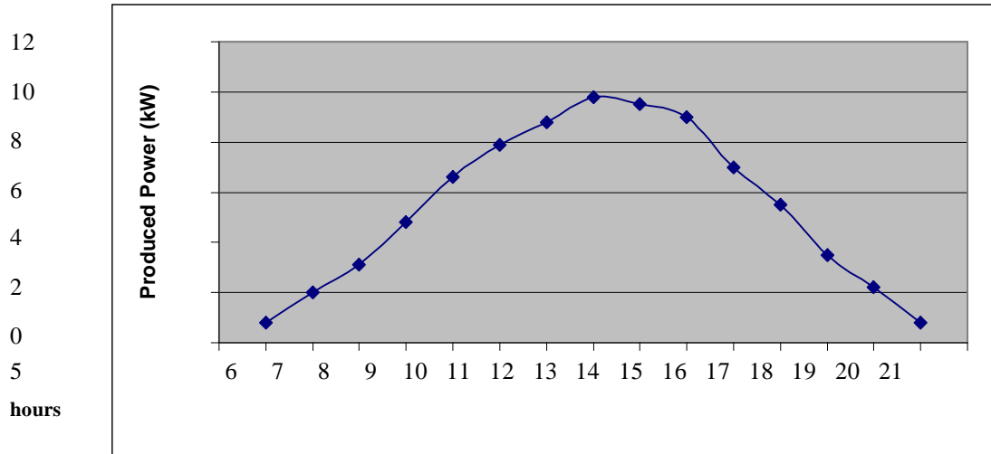
Σχήμα 7.9. Διακόμανση της μέγιστης παραγόμενης ισχύος της φωτοβολταϊκής συστοιχίας για μια τυχαία ημέρα του Αυγούστου για κάθε ώρα της ημέρας.
