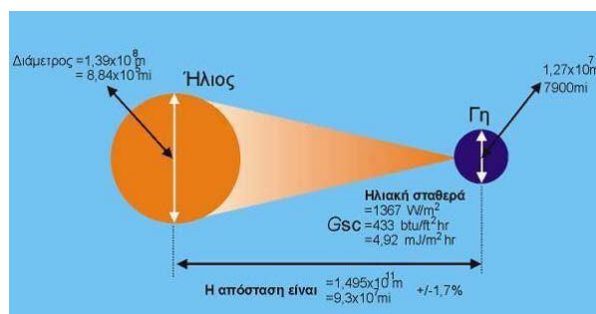
Σχήμα 2.7. Το σχήμα δείχνει σχηματικά τη γεωμετρική σχέση ήλιου-γης, η εκκεντρότητα της τροχιάς
