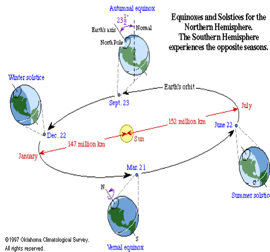
Σχήμα 2.2. Τροχιά της γης γύρω από τον ήλιο.
