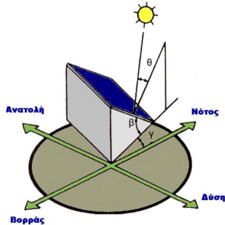
Σχήμα 2.14. Η κλίση ( \beta ) και η αζιμούθια γωνία ( \gamma ) που χαρακτηρίζουν τον προσανατολισμό ενός επίπεδου ηλιακού συλλέκτη στην επιφάνεια της γης. [9]
