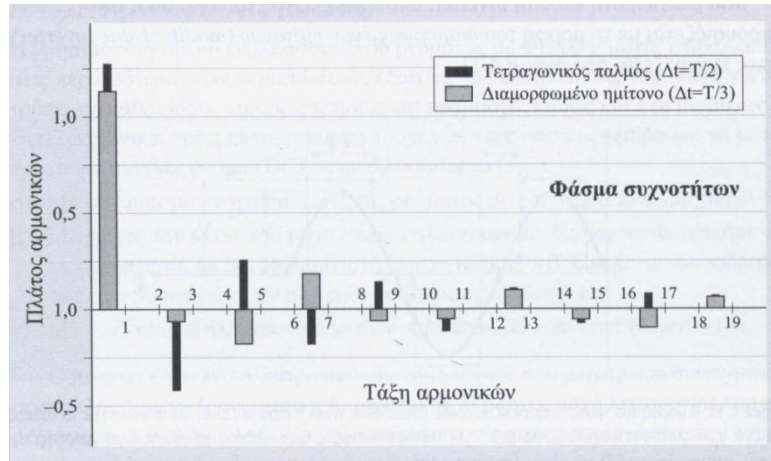
Σχήμα 5.6. Φάσμα συχνοτήτων δύο περιοδικών σημάτων, του εναλλασσόμενου τετραγωνικού παλμού (μαύρα παραλληλόγραμμα) και του εναλλασσόμενου διαμορφωμένου τετραγωνικού παλμού. Το πλάτος της θεμελιώδους αρμονικής (τάξη n=1 ) είναι \sim 1,15 του πλάτους του τετραγωνικού παλμού ( V_0 = 1,15V_p ). [8]
