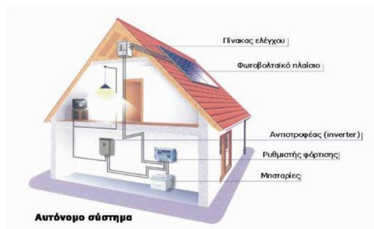
Σχήμα 1.12. Αυτόνομο Φ/Β σύστημα.
