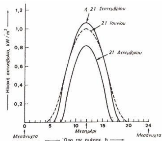
Σχήμα 2.5. Διακύμανση της έντασης της ηλιακής ακτινοβολίας με τον ηλιακό συλλέκτη σε κλίση ίση με το γεωγραφικό πλάτος του τόπου. [9]
