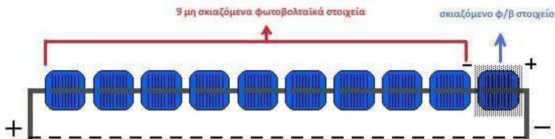
Σχήμα 3.18. Διάταξη φ/β στοιχείων σε σειρά με ένα σκιαζόμενο.
