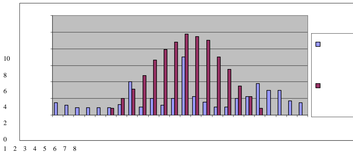
Σχήμα 7.10. Συγκριτικό ιστόγραμμα παραγόμενης ισχύος πλαισίων και καταναλισκομένης ισχύος από οικιακές συσκευές για κάθε ώρα ημέρας Αυγούστου.
