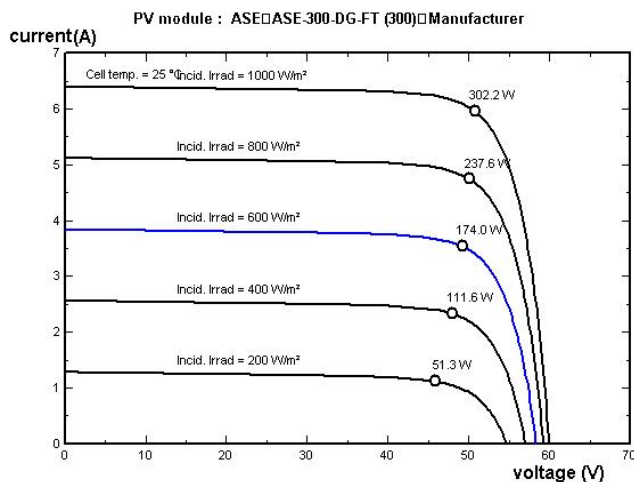
Σχήμα 3.11. Χαρακτηριστικές I - V για διάφορες τιμές της προσπίπτουσας ακτινοβολίας. Η θερμοκρασία λειτουργίας πλαισίου παραμένει σταθερή στους 25^{\circ} C . Με τη μείωση της προσπίπτουσας ακτινοβολίας παρατηρείται σημαντική μείωση του ρεύματος βραχυκύκλωσης και της παραγόμενης ισχύος στο MPP. Αντίθετα η τάση ανοιχτοκύκλωσης μεταποίζεται ελαφρά.
