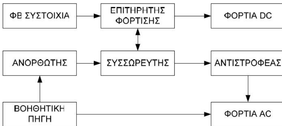
Σχήμα 1.14. Υβριδικό Φ/Β σύστημα. [8]
