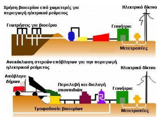
Σχήμα 1.7. Τρόπος παραγωγής βιοαερίου από χωματερές και μονάδες επεξεργασίας αστικών αποβλήτων. [27]
