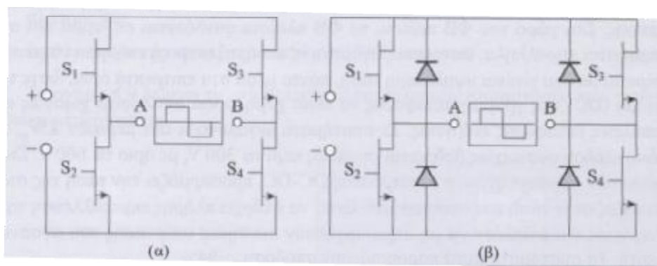
Σχήμα 5.4. (α) Βασική αρχή λειτουργίας του inverter. Τα S_1, S_2, S_3, S_4 είναι διακοπτικά στοιχεία. Η μετατροπή του συνεχούς ρεύματος σε εναλλασσόμενο (DC-AC conversion) επιτυγχάνεται με κλείσιμο-άνοιγμα των διακοπτικών στοιχείων ανά δύο, χιαστί (1,4 και 2,3). Όσο τα S_1, S_4 είναι αγώγιμα και τα S_2, S_3 σε αποκοπή, τα σημεία A και B έχουν πρόσημα + και - αντίστοιχα. Όταν συμβαίνει το αντίστροφο, τα A και B έχουν πρόσημα - και + αντίστοιχα. Με αυτόν τον τρόπο δημιουργείται η εναλλασσόμενη τετραγωνική τάση (κέντρο του διαγράμματος). (β) Στο προηγούμενο κύκλωμα προστίθεται σε κάθε διακοπτικό στοιχείο από μία δίοδο, έτσι ώστε να αποκόπτεται η επιστρεφόμενη ισχύς από μη ωμικά φορτία κατανάλωσης. [8]
