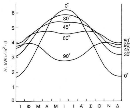
Σχήμα 2.15. Παράδειγμα της εξάρτησης της μέσης ημερήσιας ηλιακής ακτινοβολίας H_t που δέχεται μια επίπεδη επιφάνεια κατά τη διάρκεια των διαφόρων μηνών του έτους, σε συνάρτηση με την κλίση της. Το παράδειγμα είναι για τοποθεσία με γεωγραφικό πλάτος 45^\circ και αφορά σε κλίσεις του ηλιακού συλλέκτη ίσες με 0^\circ (οριζόντιο επίπεδο), 30^\circ , 45^\circ , 60^\circ και 90^\circ (κατακόρυφο επίπεδο). [9]
