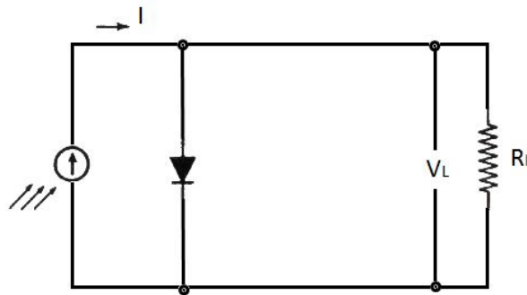
Σχήμα 3.7. Ιδανικό ισοδύναμο ηλεκτρικό κύκλωμα ενός Φ/Β στοιχείου. [9]
