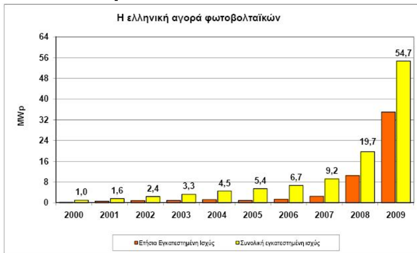
Σχήμα 1.8. Εξέλιξη της εγκατεστημένης ισχύος των φωτοβολταϊκών στην Ελλάδα. [28]
