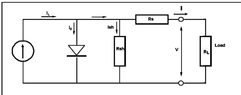
Σχήμα 3.8. Το ισodύναμο ηλεκτρικό κύκλωμα ενός Φ/Β στοιχείου που περιλαμβάνει τις αντιστάσεις σειράς R_s , καθώς και τις παράλληλες αντιστάσεις R_{sh} . [9]
