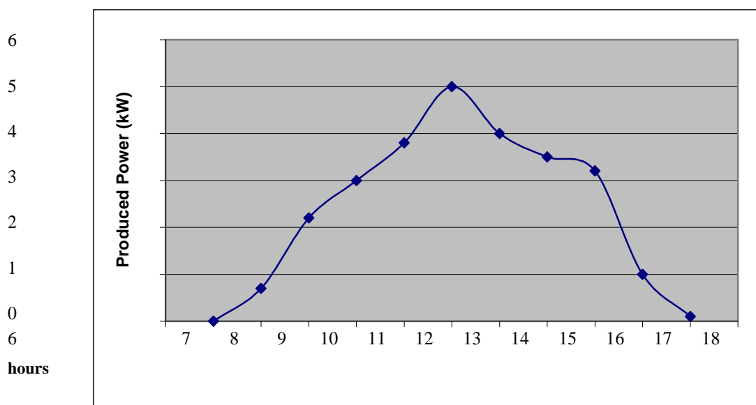
Σχήμα 7.7. Διακύμανση της μέγιστης παραγόμενης ισχύος της φωτοβολταϊκής συστοιχίας για μια τυχαία ημέρα του Δεκεμβρίου για κάθε ώρα της ημέρας.
