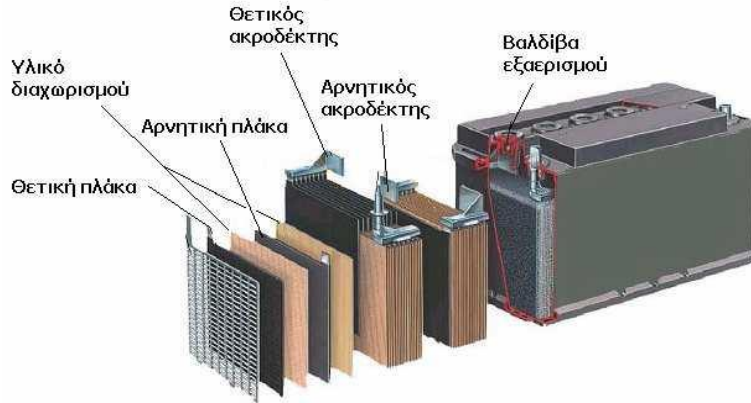
Σχήμα 4.2. Η δομή ενός συσσωρευτή.
