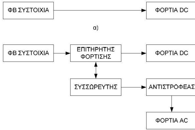
Σχήμα 1.13. Αυτόνομο Φ/Β σύστημα α) άμεσης τροφοδοσίας του φορτίου και β) με αποθήκευση της παραγόμενης ενέργειας. [8]
