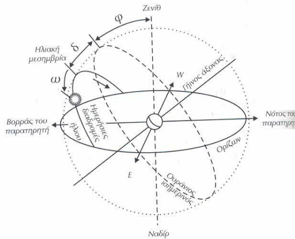
Σχήμα 2.10. Το τοπικό σύστημα συντεταγμένων Ζενίθ- Ναδίρ που δείχνει τη φαινόμενη ημερήσια κίνηση του ήλιου.
