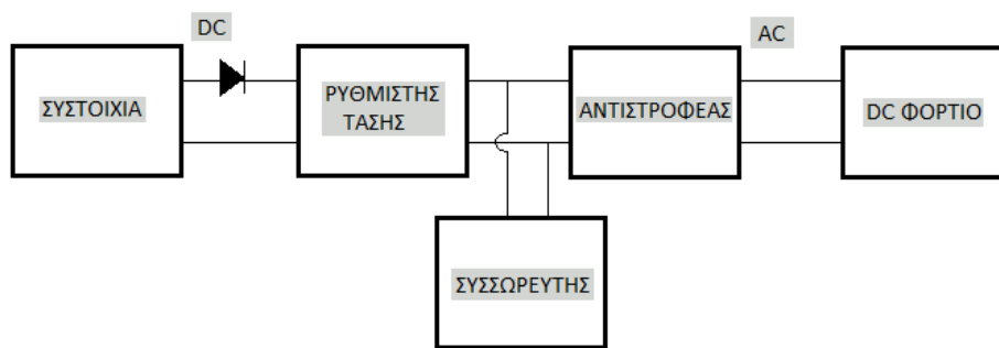
Σχήμα 5.3. Φωτοβολταϊκό σύστημα με αντιστροφή. [24]
