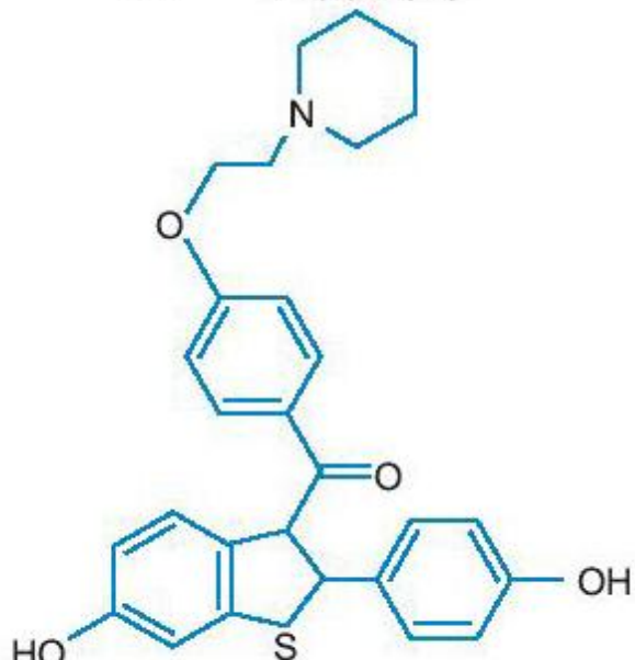
Raloxifene
