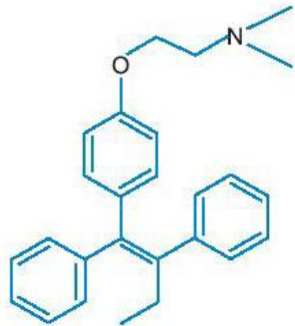
Tamoxifen
