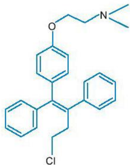
Toremifene
