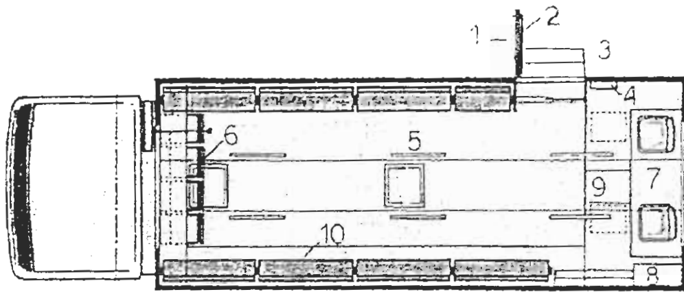
Σχήμα Δ: (1) Είσοδος και Έξοδος. (2) Χειρολαβή προσαρμοσμένη στην πόρτα. (3) Σκαλοπάτι που αναδιπλώνεται κάτω από το σασί. (4) Ηλεκτρικός πίνακας. (5) Λάμπα φθορίου. (6) Θήκες για άλμπουμ. (7) Οθόνη προβολής. (8) Ντουλάπα για φύλαξη παλτών. (9) Γραφείο δανεισμού. (10) Χαμηλά ντουλάπια με πόρτες που σκεπάζουν.
