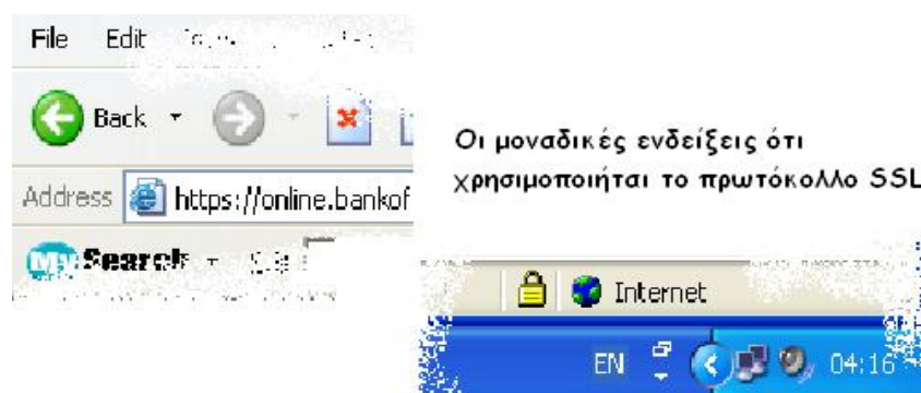
Εικόνα 13:Πρωτόκολλο SSL
