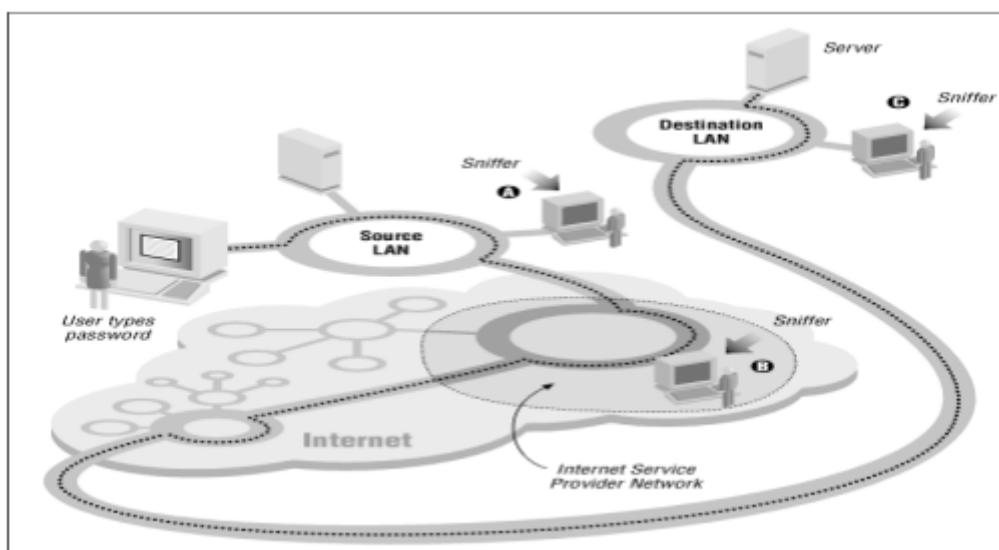
Εικόνα 6:sniffers
