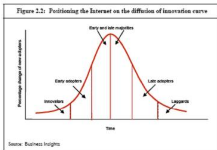
Εικόνα 3: Καμπύλη καινοτομίας
