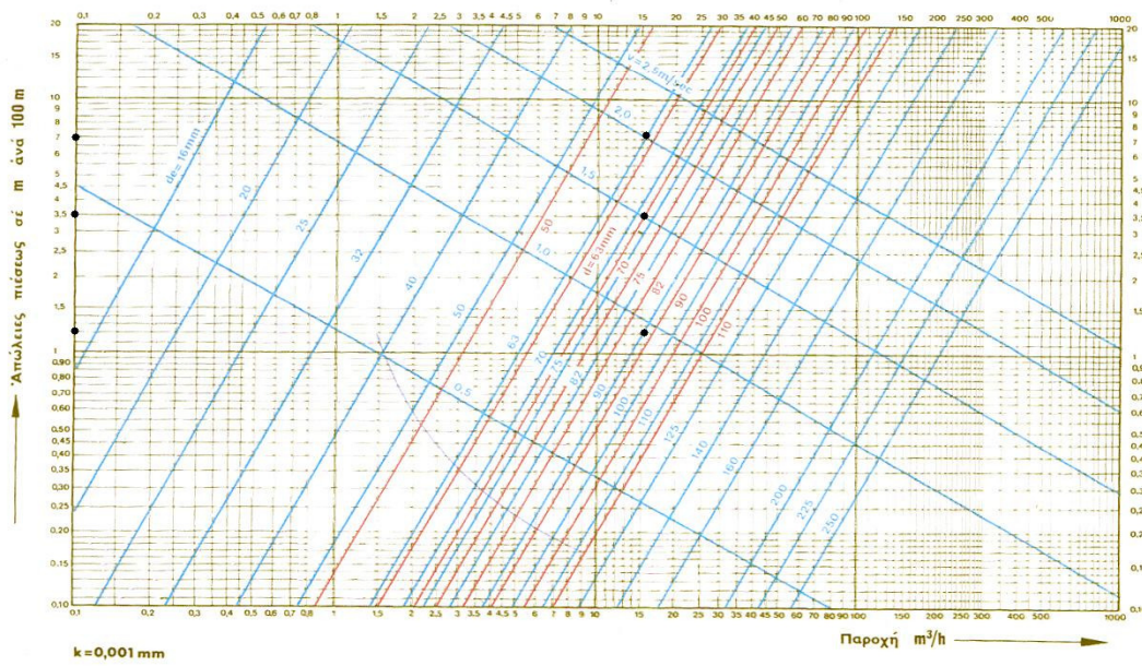
Πίνακας 4. Νομογράφημα απωλειών πιέσεων σωλήνων P.E. 10 Atm.
