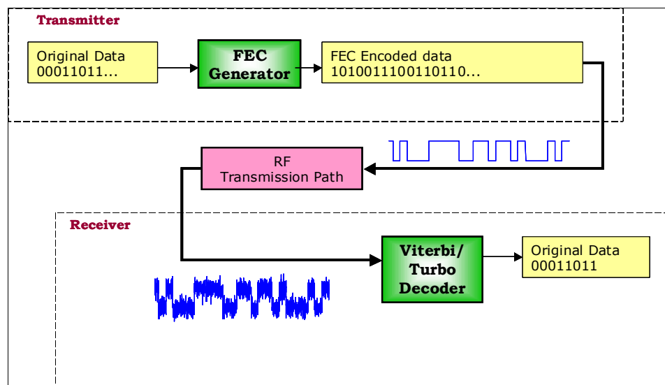
Σχήμα 4.8 : Κωδικοποίηση FEC: Ο συνελικτικός κωδικοποιητής
