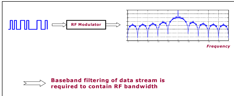
Σχήμα 6.5: Φιλτράρισμα δεδομένων.
