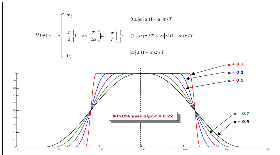
Σχήμα 6.7: Raised-Cosine Δεδομένα φίλτρου, Εξισώσεις
