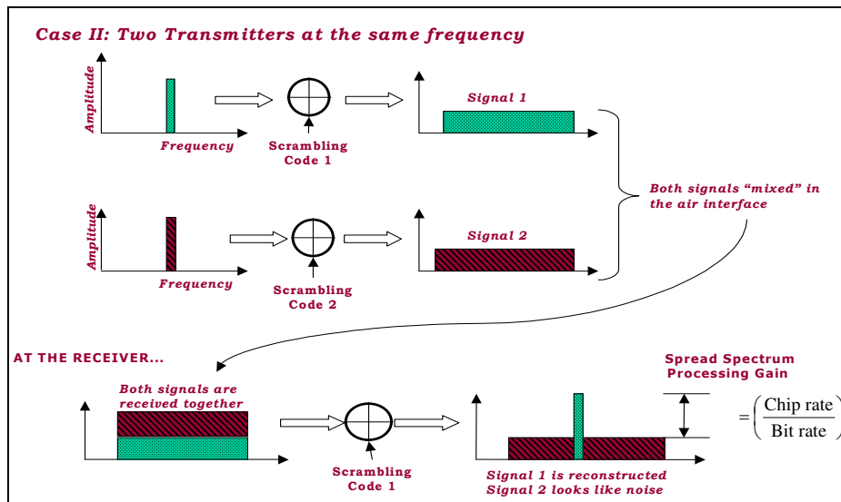
Σχήμα 5.3: Δύο πομποί με την ίδια συχνότητα
