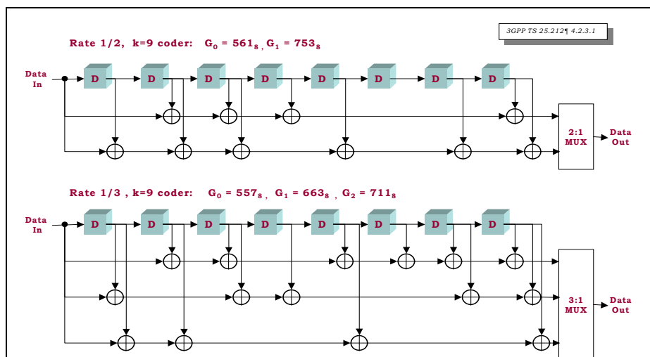
Σχήμα 4.11: Συνελκτικές γεννήτριες κώδικα
