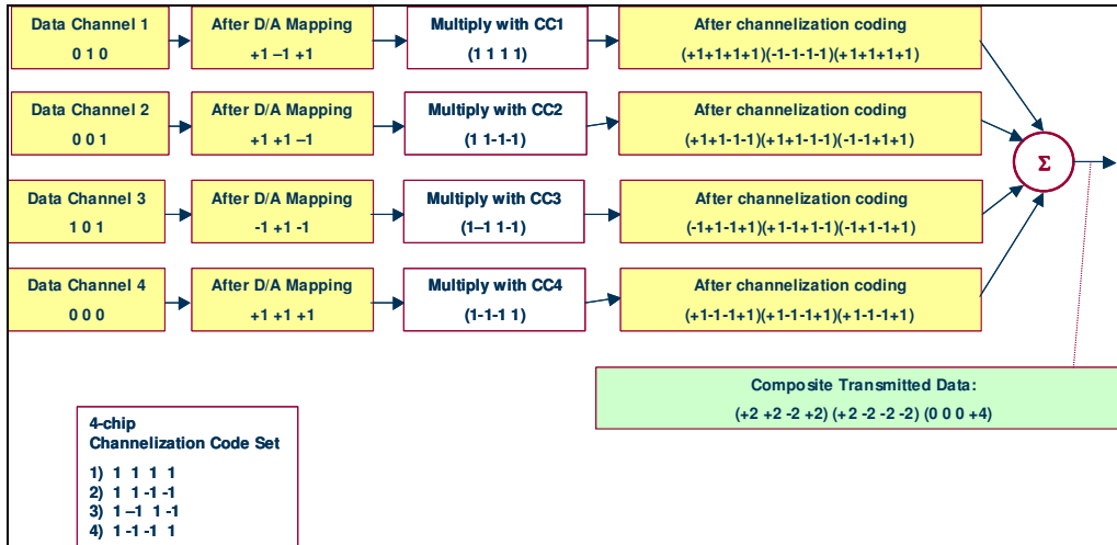
Σχήμα 4.27: Κωδικοποίηση Channelization παράδειγμα - πομπού.
