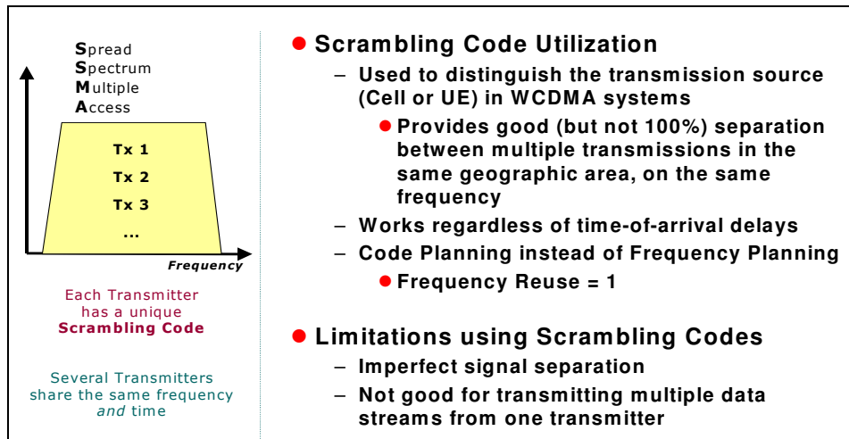
Σχήμα 5.9: Περίληψη Κωδικού κρυπτογράφησης
