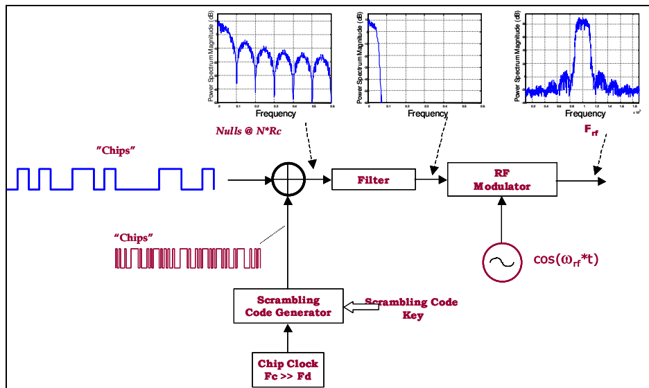
Σχήμα 5.3: Γιατί ονομάζεται διασκορπισμένου φάσματος;
