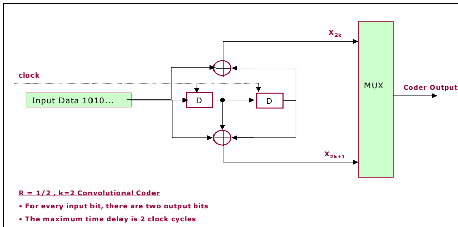
Σχήμα 4.9: Παράδειγμασυνελικτικής κωδικοποίησης.
