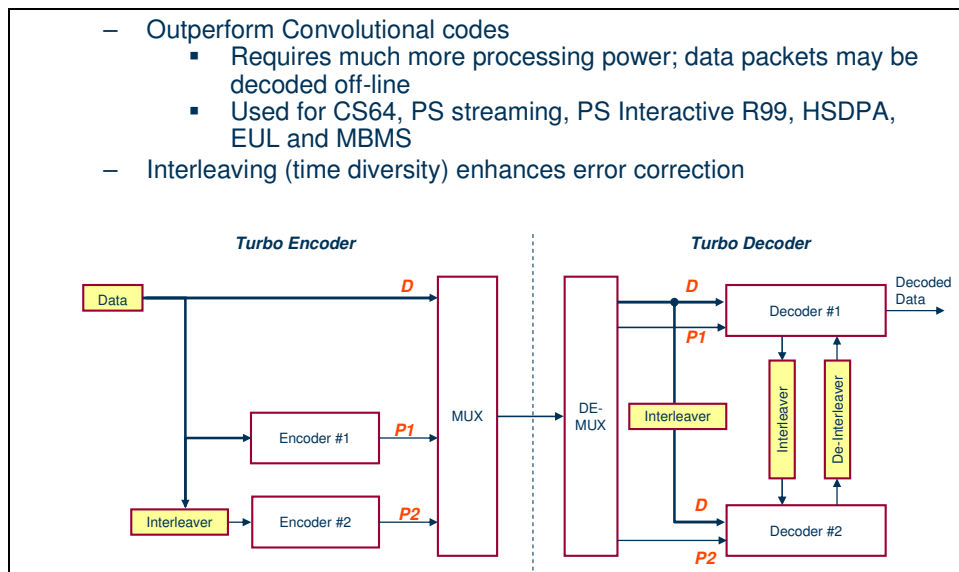
Σχήμα 4.19: Turbo Κωδικοποίηση.
