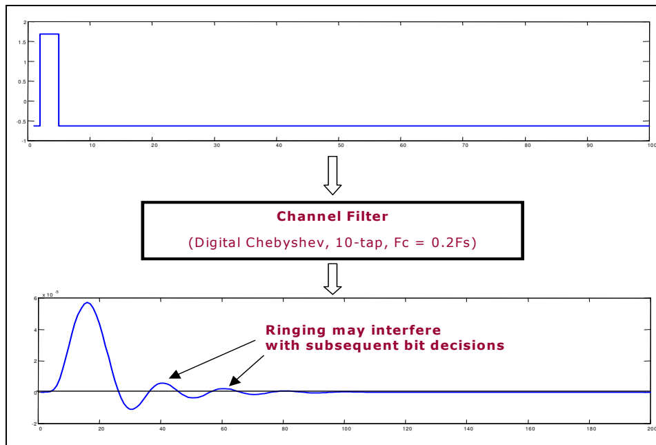
Σχήμα 6.6: φιλτράρισμα δεδομένων, σύνθετος Φίλτρο Καναλιού: Κρουστική Απόκριση
