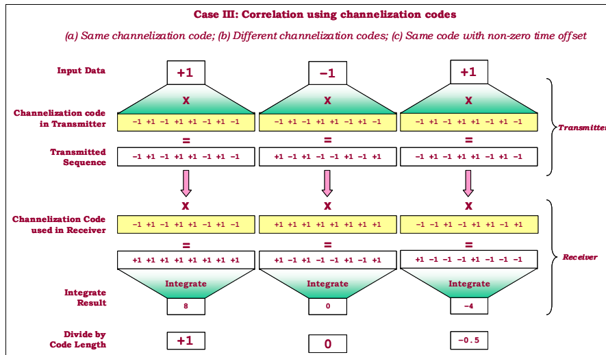
Σχήμα 4.23: αντιστοίχιση κωδικού: Συσχέτιση χρήση κωδικών Channelization
