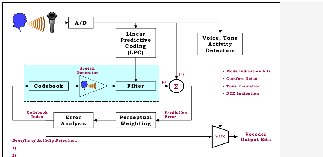
Σχήμα 3.5: ACELP Voice Coding
