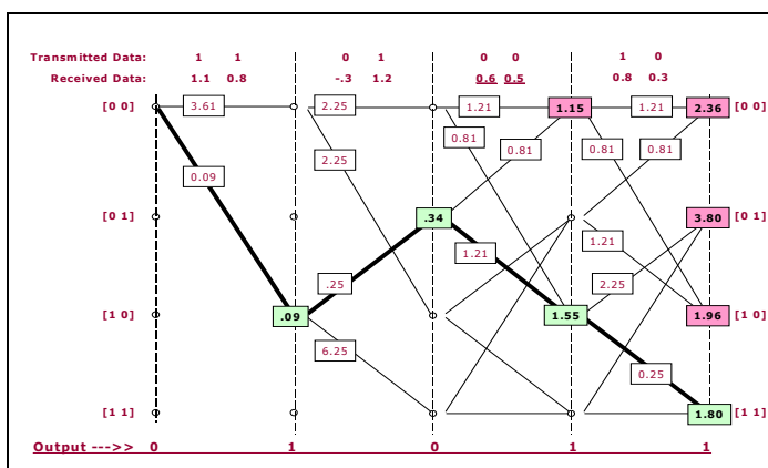
Σχήμα 4.14: Viterbi αποκωδικοποίησης, με θόρυβο.
