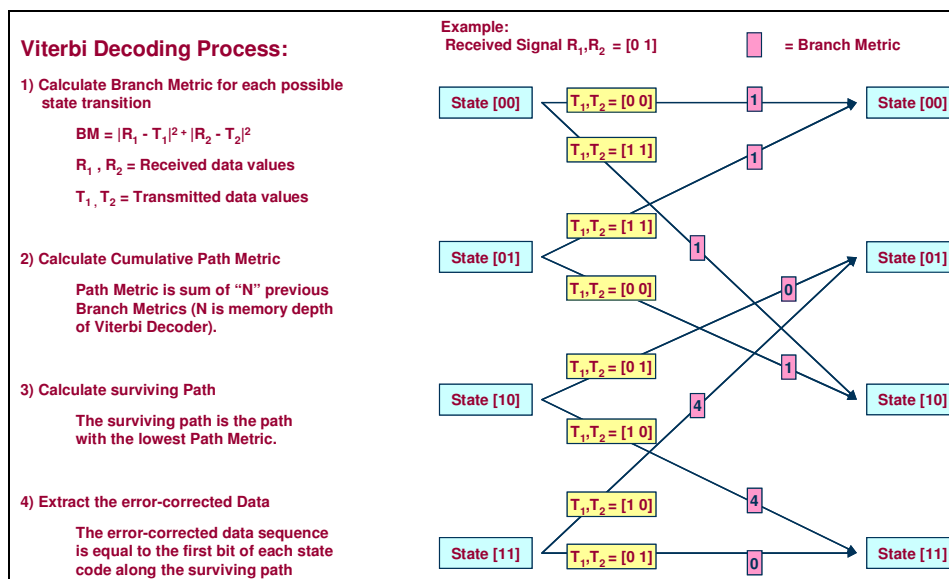
Σχήμα 4.12: Viterbi αποκωδικοποιητής
