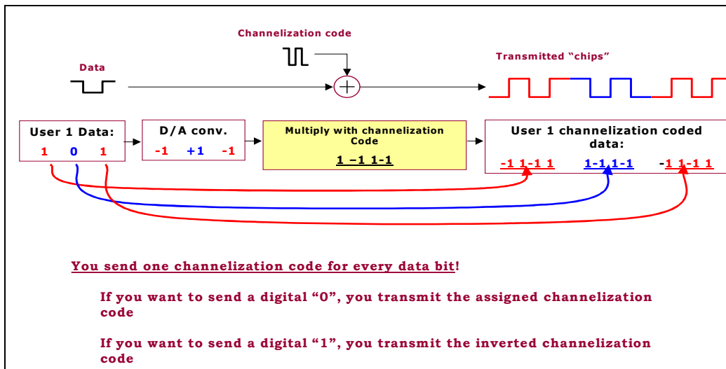
Σχήμα 4.26: Κωδικοί Channelization.
