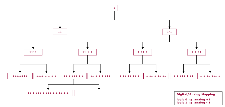
Σχήμα 4.30 : Δημιουργία Channelization κώδικα.
