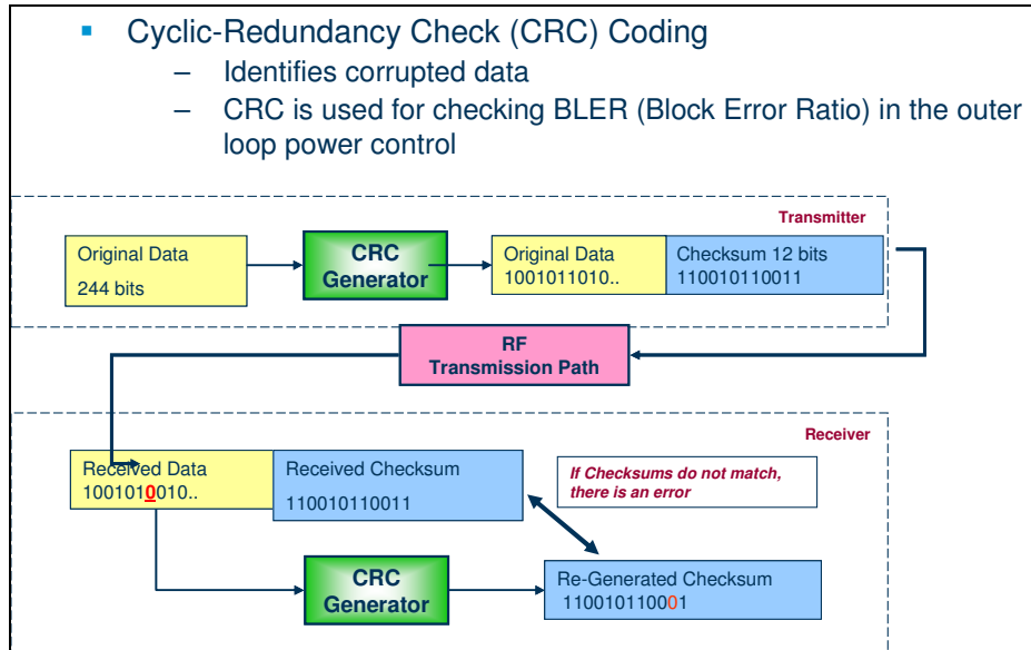
Σχήμα 4.3: CRC Coding
