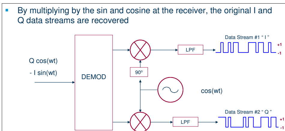
Σχήμα 6.3: I / Q Αποδιαμόρφωση - πολλαπλασιάζοντας το ημίτονο και το συνημίτονο στο δέκτη, ανακτώνται οι αρχικές I και Q ροές δεδομένων.
