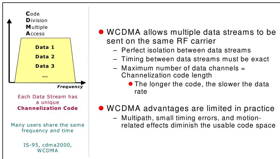
Σχήμα 4.33 Περίληψη των Κωδικών Channelization
