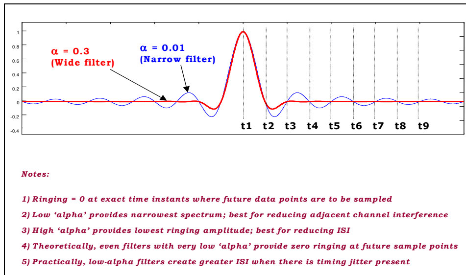
Σχήμα 6.8: Raised-Cosine δεδομένων Φίλτρου: Κρουστική Απόκριση
