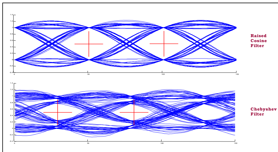
Σχήμα 6.9: Σύγκριση Διαγραμμάτων «ματιού» μεταξύ Raised-CosineDataFilter και ChebyshevFilter.
