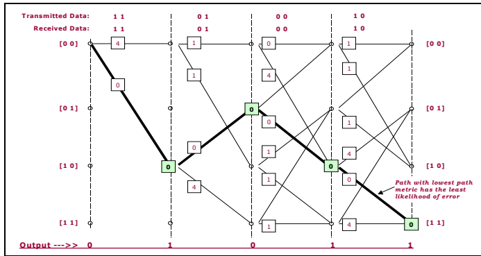
Σχήμα 4.13: Viterbi αποκωδικοποίηση, χωρίς θόρυβο
