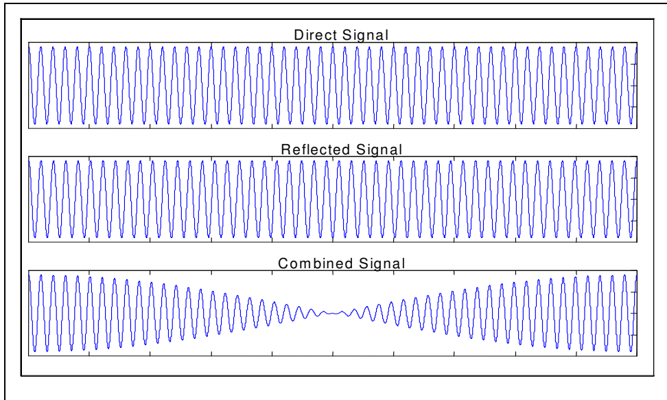
Σχήμα 4.16: εξασθένηση πολλαπλών διαδρομών.
