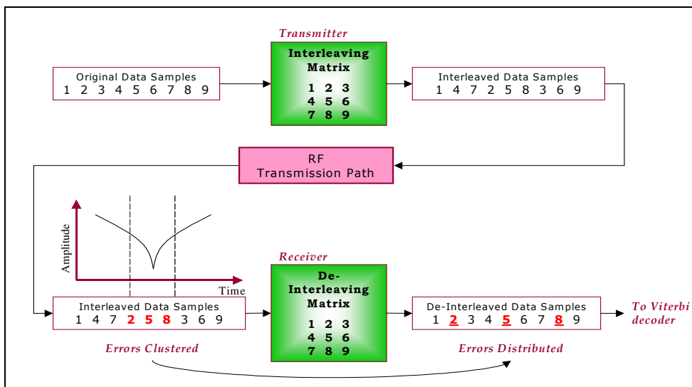
Σχήμα 4.17 :BlockInterleaving.
