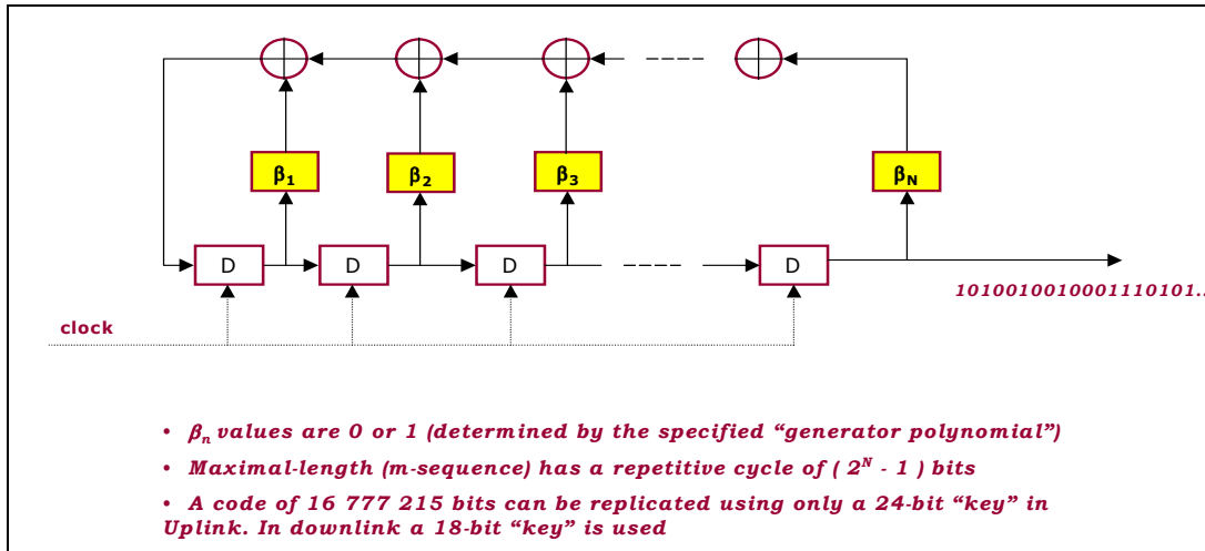
Σχήμα 5.6: Δημιουργία κώδικα κρυπτογράφησης
