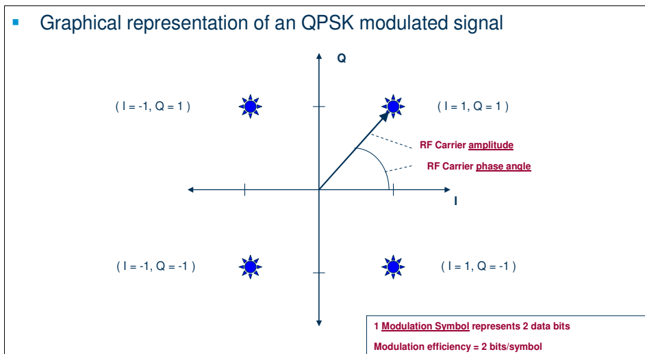
Σχήμα 6.2: Διαμόρφωση QPSK - γραφική αναπαράσταση μιας μονάδας I / Q διαμορφωμένου σήματος.
