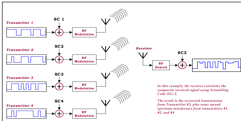
Σχήμα 5.2 Spread Spectrum Multiple Access
