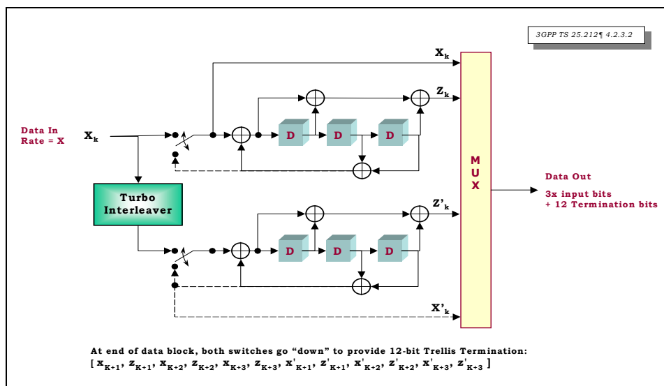
Σχήμα 4.20 : WCDMA γεννήτρια Turbo κώδικα
