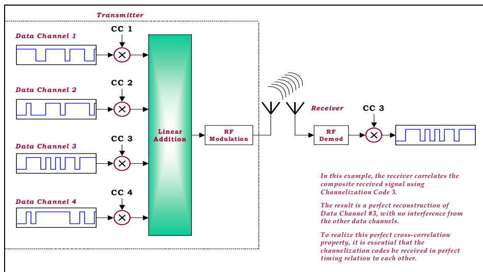
Σχήμα 4.25: κωδικοποίηση Channelization
