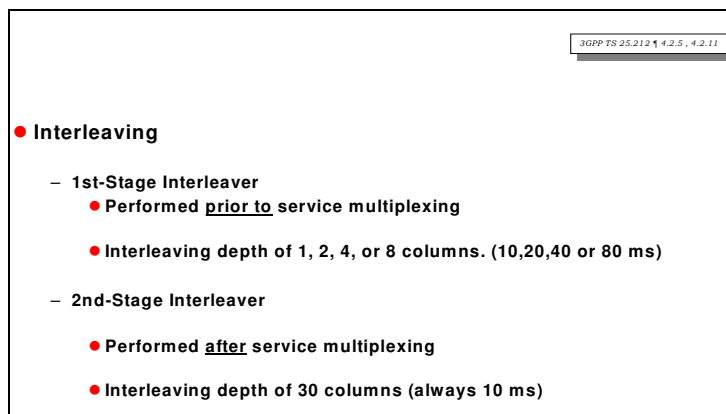
Σχήμα 4.18 : 1ο και 2 ο interleaver
