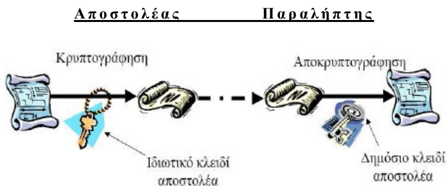
Εικόνα 10: Κρυπτογραφικό σύστημα δημόσιου κλειδιού
