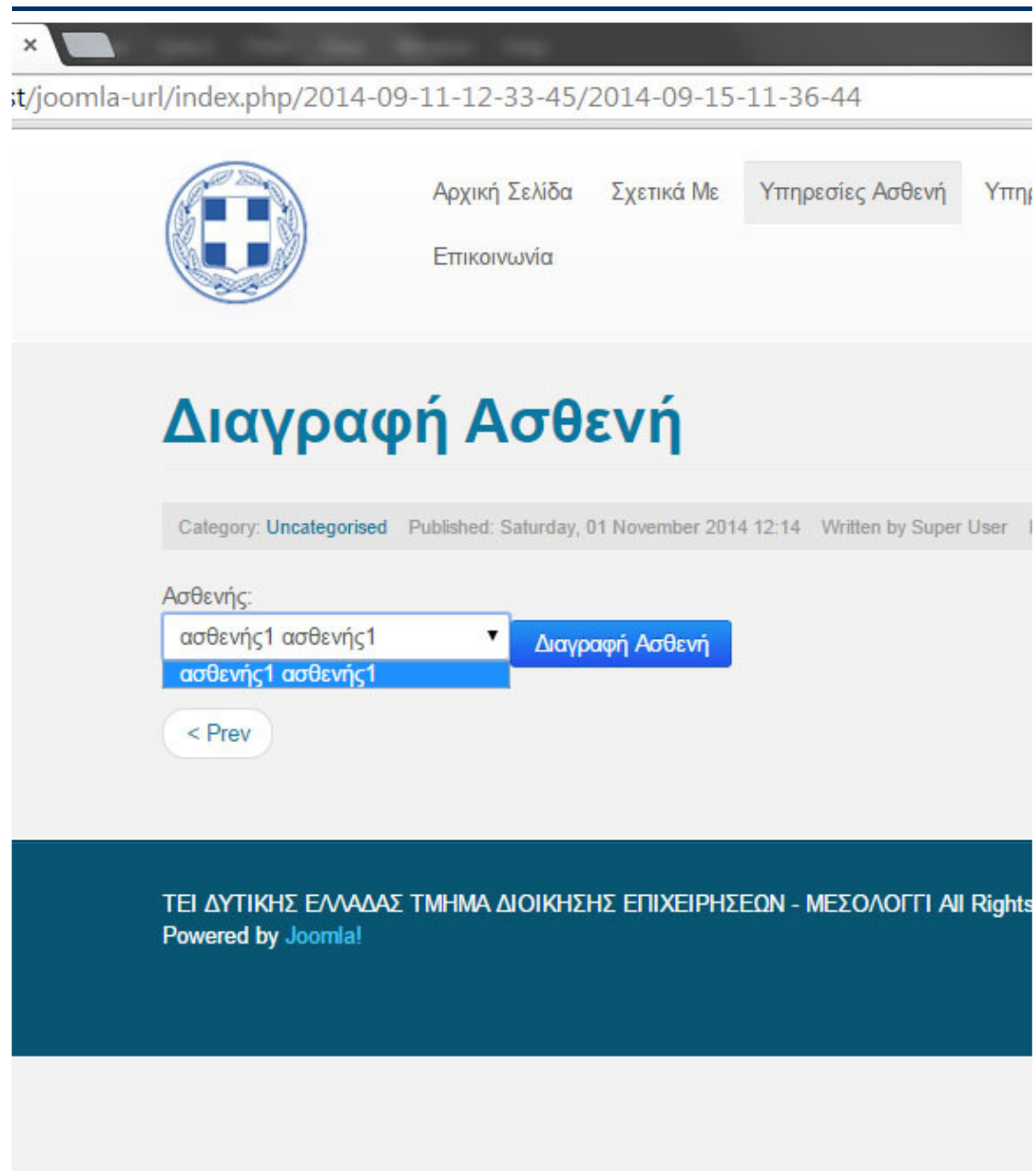
Εικόνα 28: Φόρμα Διαγραφής Ασθενή
