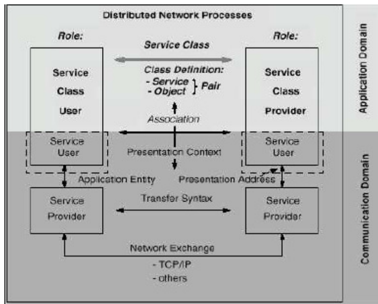
Εικόνα 7: Αρχές λειτουργίας DICOM σε δίκτυο
