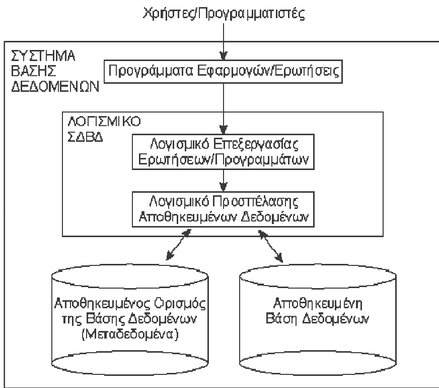
Εικόνα 11: Σύστημα Βάσης Δεδομένων
